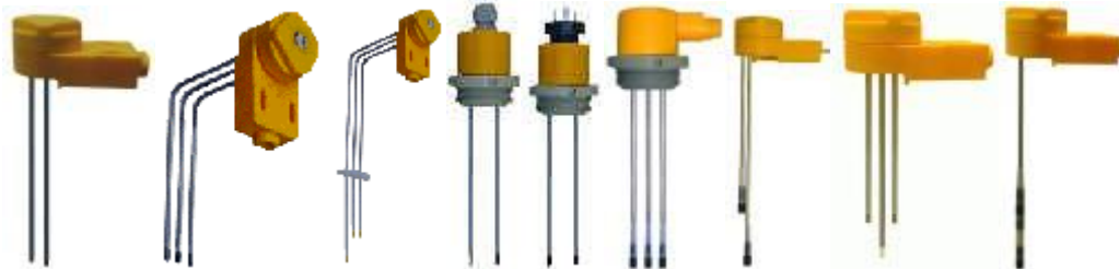
Trockenheizschutz / Niveau-Metall-Teflon-Stabelektroden mit oder ohne PT 100, PTC-Fühler integrierter Stromschleife, Analog-Linear Temperatur/Spannungswandler usw.
